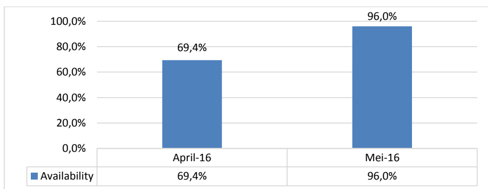
Gambar 5. Hasil Improvement Availability (April dan Mei 2016)
