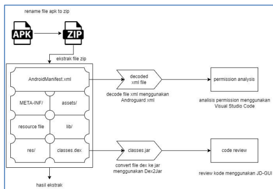
Gambar 10. Alur Proses Decompile Aplikasi
