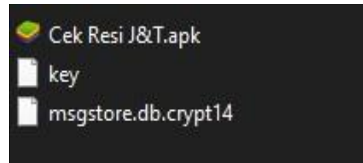
Gambar 6. Hasil Ekstraksi
