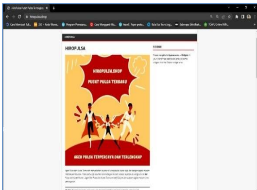
Gambar 15. Website Mencurigakan
