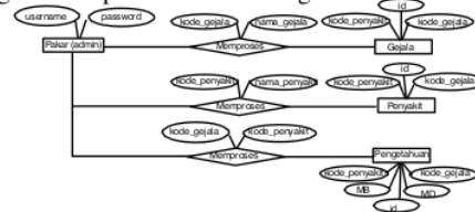
Gambar 2. Diagram entitas antar atribut
