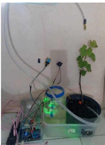
Gambar 5. Prototipe Sistem
