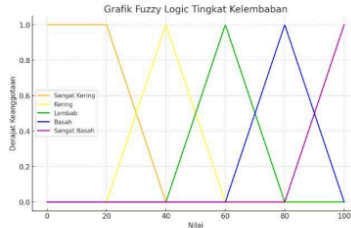
Gambar 2. Grafik Fuzzy Kelembapan Tanah
