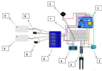
Gambar 1. Rangkaian Sistem
