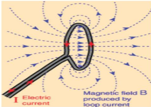
Gambar 5. Medan magnet pada kawat loop . Sumber: Suyoso, 2003.
