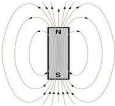
Gambar 6. Medan magnet pada magnet batang. Sumber: Suyoso, 2003.
