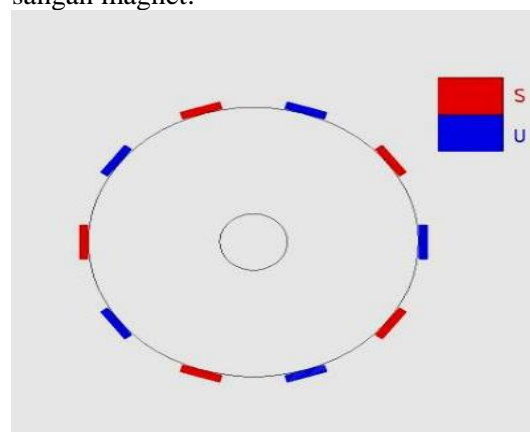
Gambar 19. Posisi Pemasangan Magnet.
