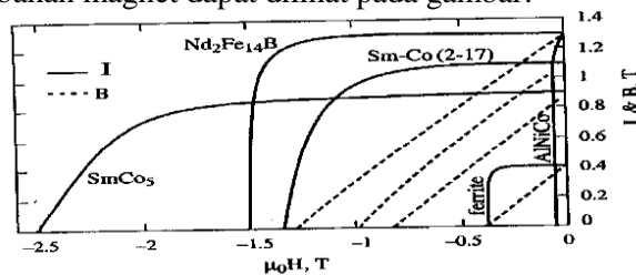
Gambar 18. Kurva karakteristik magnetik beberapa material magnet permanen.
