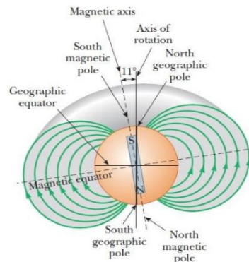
Gambar 8. Medan magnet pada bumi Sumber: Suyoso, 2003.
