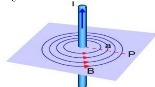
Gambar 4. Garis Medan Magnet Pada Kawat Lurus. Sumber: Suyoso, 2003.
