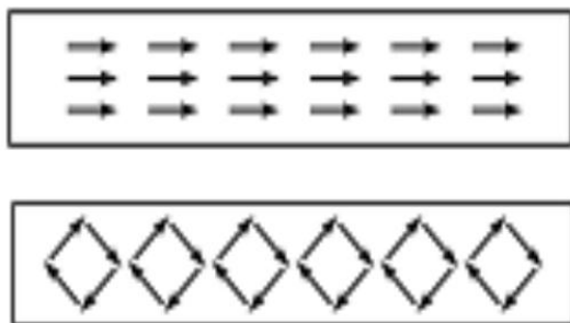
Gambar 2. Susunan magnet elementer besi/baja sebelum dan sesudah menjadi magnet. Sumber: Suyoso, 2003.
