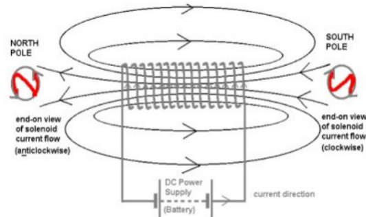
Gambar 7. Medan magnet pada solenoid. Sumber: Suyoso, 2003.
