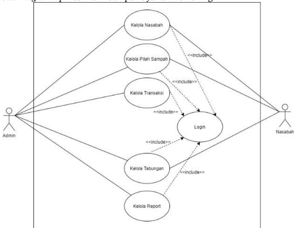
Gambar 4 Use Case Diagram Aplikasi Bank Sampah Syariah Kemuning
