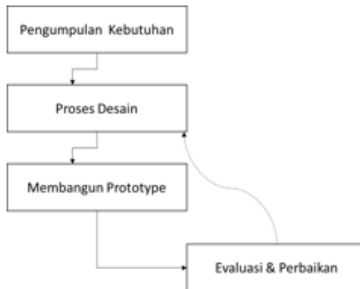
Gambar 1 Langkah-Langkah Prototyping
