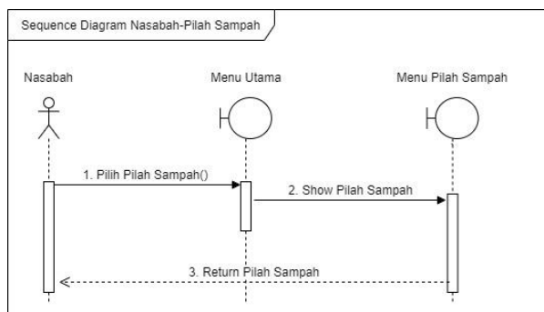
Gambar 6 Sequence Diagram Pilih Sampah
