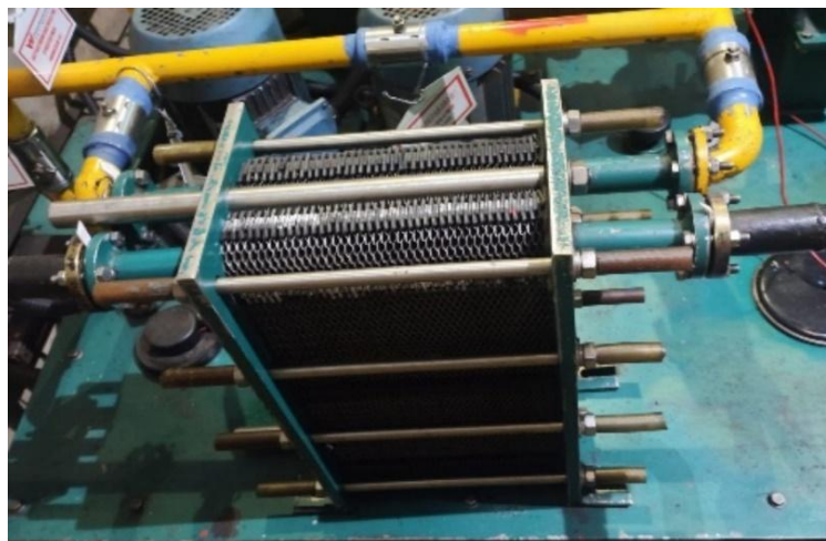
Gambar 1. Heat Exchanger Tipe Plat Model BR015-4 pada Sistem Pompa Feedwater PLTU 4 x 25 MW.
