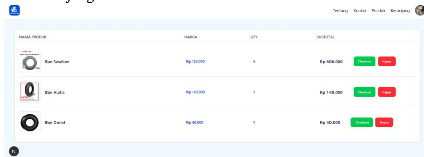
Gambar 6 Halaman Keranjang
