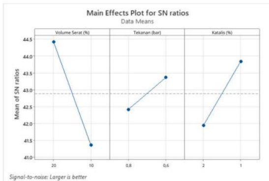
Gambar 6. Rasio S/N
