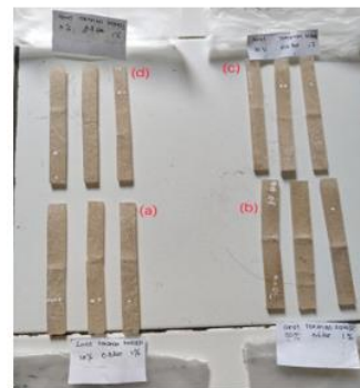
Gambar 5. Sampel biokomposit setelah diuji bending (a) variasi 1, (b) variasi 2, (c) variasi 3, (d) variasi 4
