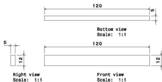
Gambar 2. Standar benda uji bending standar ASTM-D 790
