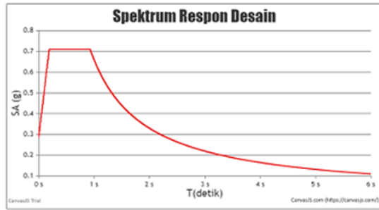
Gambar 6. Hasil Spektrum Respons Desain Bangunan dari Data Puskim (SE)
