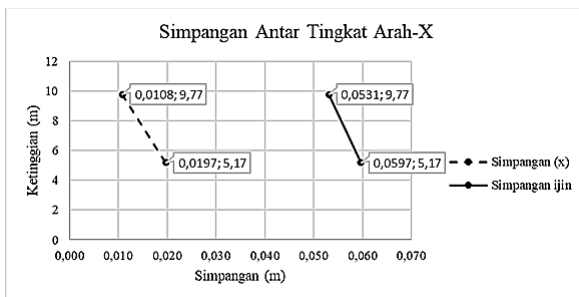
Gambar 8. Simpangan Antar Tingkat Arah-x (K2)
