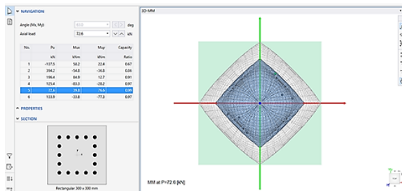
Gambar 12. Kapasitas Kolom K2
