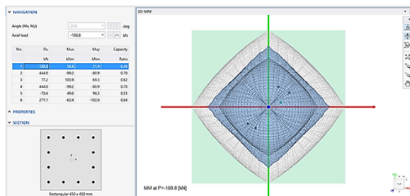
Gambar 11. Kapasitas Kolom K1
