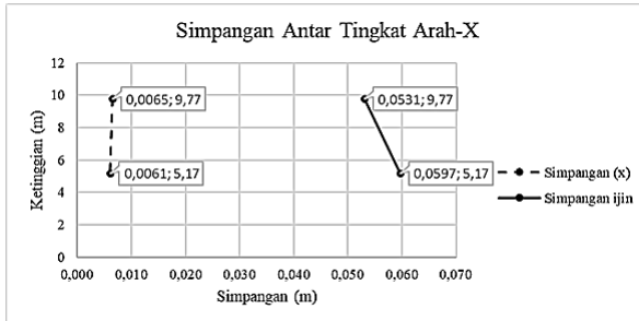
Gambar 7. Simpangan Antar Tingkat Arah-x (K1)
