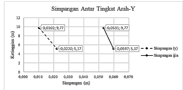
Gambar 10. Simpangan Antar Tingkat Arah-y (K2)
