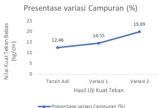
Gambar 4. Grafik hasil pengujian kuat tekan bebas (hasil analisis)
