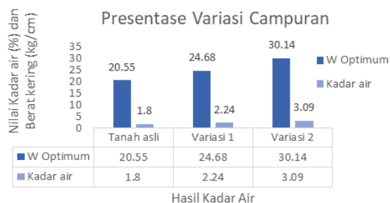
Gambar 3. Grafik Hasil Uji Pemadatan (Proctor Standard) (hasil analisis)
